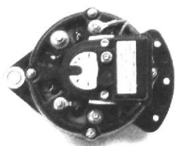
ALTERNADOR 65 AMP. 30-50324-00
