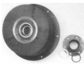
EMBRAGUE UNIDAD REMOLQUE CUBO ENSAMBLADO 50-00225-03
